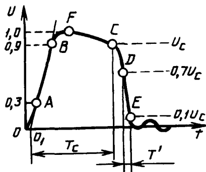
Рисунок 9 — Грозовой импульс, срезанный на спаде импульса
