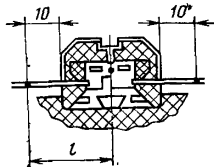
к наборному зажиму однопроволочной жилы*
