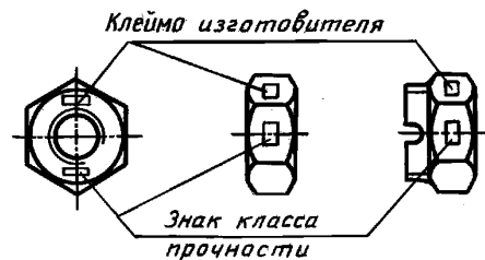
Черт. 2
