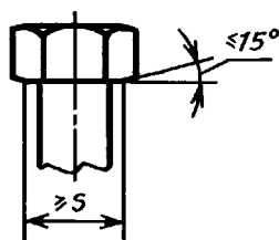
Черт. 5
