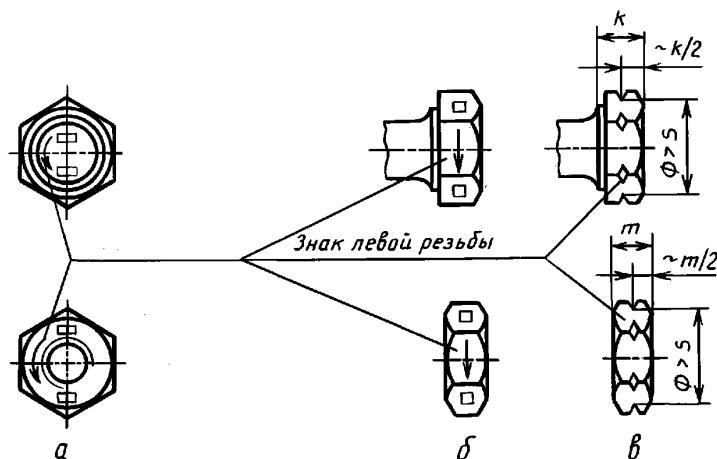
Черт. 4
