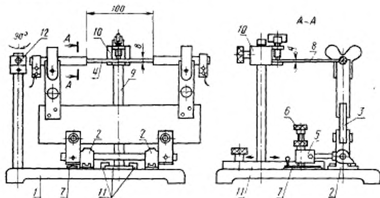
1—плоская плита 2—поддвижки; 3—держатель; 4—накаливаемый стержень; 5—протектор; 6—отсчетный зонг; 7—сопорогизм вращающаяся; 8—испытуемый образец; 9—держатель образца; 10—шажки 11—подвижное основание; 12—поворотный металлический стержень
