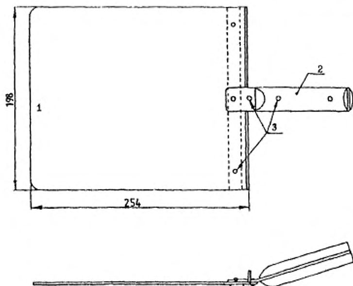
1 — плоский лист из алюминия или нержавеющей стали (толщина 2 мм); 2 — рукоятка; 3 — заплески
