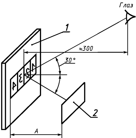
1 — образец; 2 — пластина с сеткой или рисунком; A — максимальное расстояние, при котором сетка или рисунок четко отражается на поверхности покрытия
